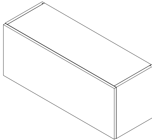
V3-90-1K LHW-900X360X320
