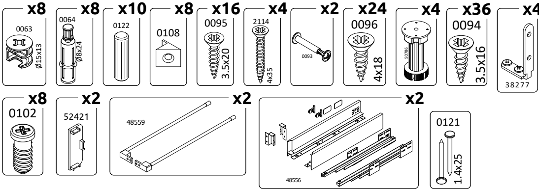
R-80-2MBOX LHW-800X943X600
