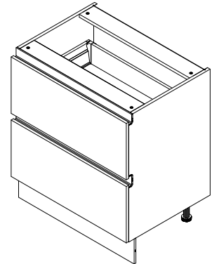
R-80-2MBOX LHW-800X943X600
