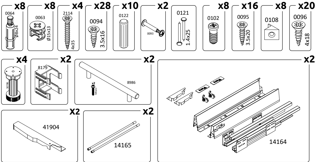
R-80-2MBOX LHW-800X870X600
