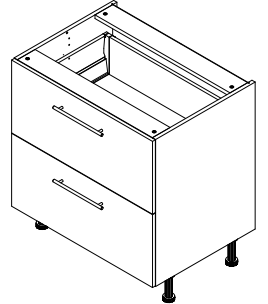
R-80-2MBOX LHW-800X870X600
